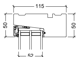
Overkarm
