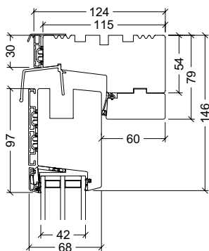
Overkarm, hæveskydedør
