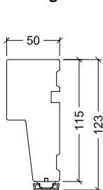
123mm karm
