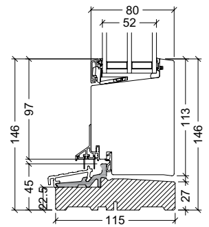
45mm hårdtræsbundkarm, indadgående dør
