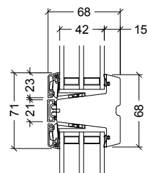
68mm gennemgående sprosse til hæveskyde- dør
