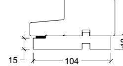
Påforing type 18-104
