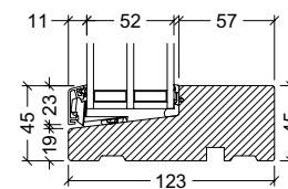
Bundkarm til fast sideparti
