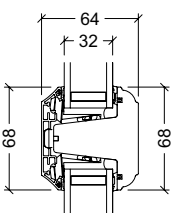
Classic alu 68mm gennemgående sprosse, 2-lags rude
