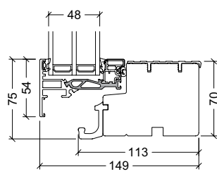
70mm bundkarm m/alu- slidskinne, skydedør
