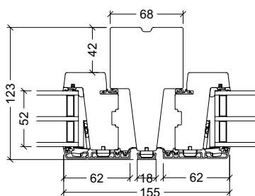
Lodpost, gående rammer Fast eller gående post
