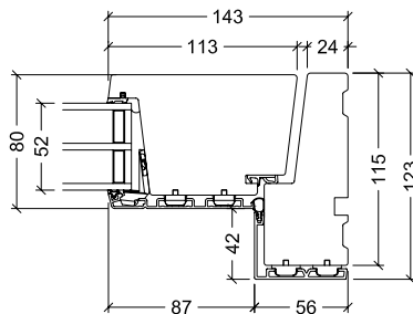
Sidekarm, indadgående dør
