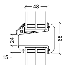
Classic træ 68mm gennemgående sprosse, 3-lags rude
