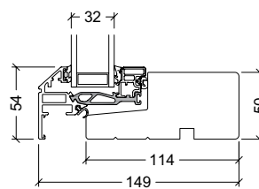
Bundkarm
