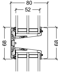
68mm gennemgående sprosse, 3-lags rude (se døre ovenfor)
