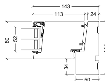
Sidekarm VELFAC Ribo trædør
