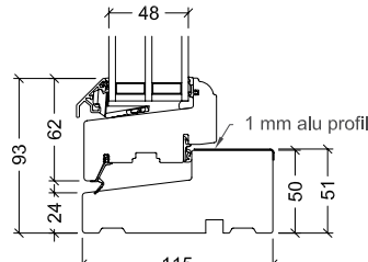
50mm bundkarm med alu-slidskinne, terrassedør (vinduesdør)
