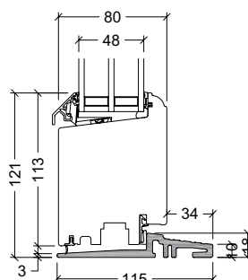
18mm HELO® bundkarm, udadgående dør OBS: 22,5mm ved 148mm karm
