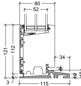
18mm HELO® bundkarm, udadgående dør OBS: 22,5mm ved 148mm karm
