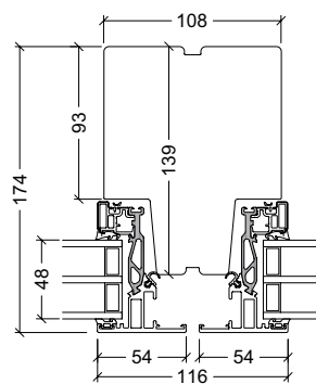
139mm lodpost (tværpost)
