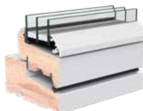
Gående element – 3-lags rude Bundkarm med aluglasliste
