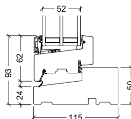
Bundkarm, gående ramme samt fastskruet ramme
