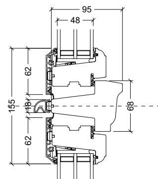
Tværpost, gående rammer
