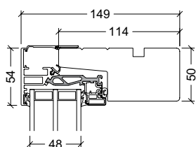
Overkarm
