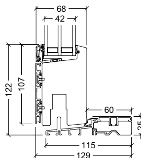
Bundkarm, hæveskydedør
