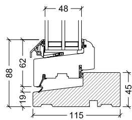
45mm hårdtræs bundkarm, terrassedør (vinduesdør)
