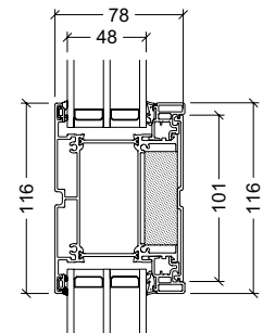
116mm gennemgående sprosse 3-lags rude
