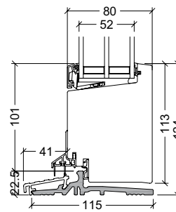
22,5mm HELO® bundkarm, indadgående dør
