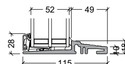
Bundkarm til fast sideparti
