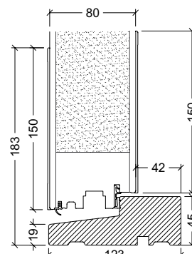
45mm hårdtræsbundkarm
