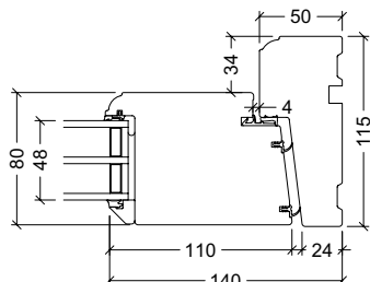
Sidekarm, udadgående dør
