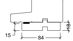
Påforing type 18-84 Også til skydedøre
