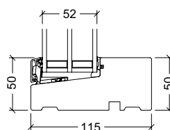
Bundkarm
