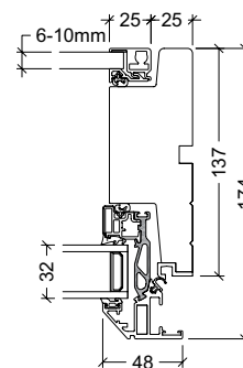
139mm karm med forsatsramme til vendevindue med 48mm rammeprofil
