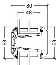
Classic alu 68mm gennemgående sprosse, 3-lags rude
