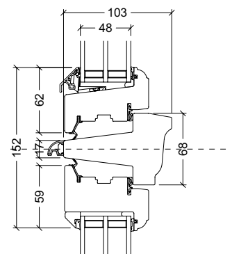
Tværpost, gående rammer
