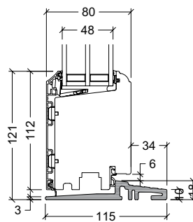
18mm HELO® bundkarm, udadgående dør OBS: 22,5mm ved 148mm karm
