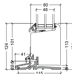
22,5mm HELO® bundkarm, indadgående dør
