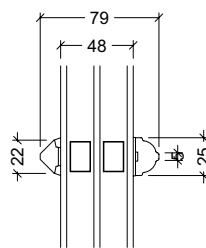
Classic træ 25mm energisprosse 3-lags rude
