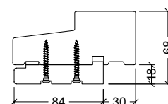
Påforing type 18x84
