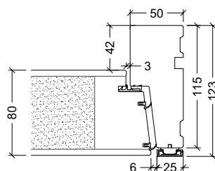
Sidekarm
