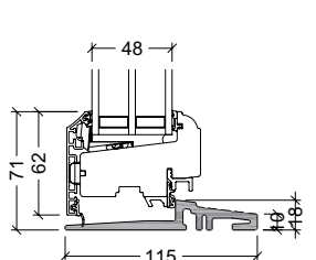
18mm HELO® bundkarm, terrassedør (vinduesdør) OBS: 22,5mm ved 148mm karm
