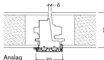
Bundkarm til fast sideparti
