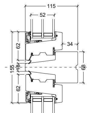
Tværpst, gående rammer
