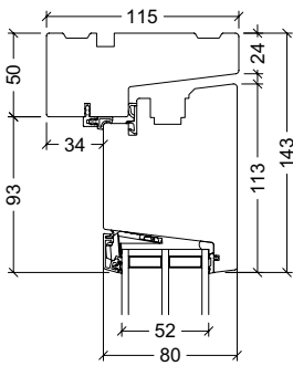
Overkarm, indadgående dør
