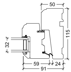
Eksempel på vindue med 2-lags rude
