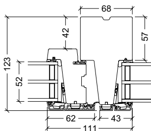
Kombinationslodpost
