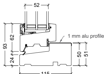
50mm bundkarm med alu-slidskinne, terrasedør (vinduesdør)
