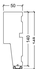
148mm karm
