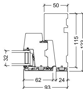
Eksempel på vindue med 2-lags rude
