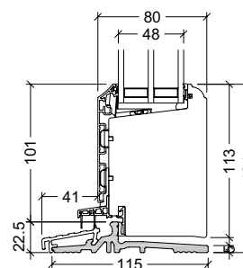
22,5mm HELO® bundkarm, indadgående dør
