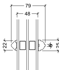
Classic træ 25mm energisprosse 3-lags rude
