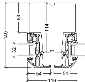
114mm lodpost (tværpost)
