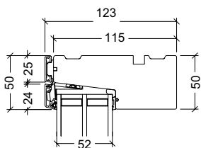
Overkarm
