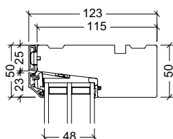
Overkarm
