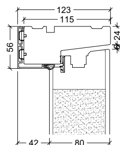
Overkarm
