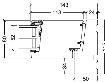
Sidekarm, indadgående dør
