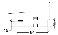
Påføring type 18-84 Også til skydedøre
