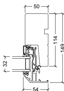
Sidekarm
