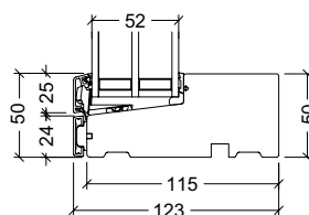
Bundkarm
