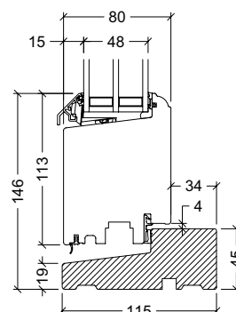
45mm hårdtræsbundkarm, udadgående dør
