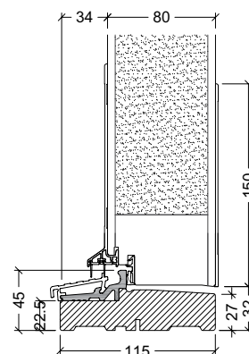
45mm hårdtræsbundkarm
