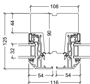
90mm lodpost (kun til vinduer)
