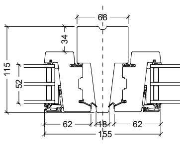
Lodpost, gående rammer Fast eller gående post
