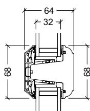
Classic alu 68mm gennemgående sprosse, 2-lags rude
