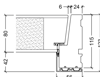
Sidekarm
