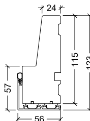
123mm karm
