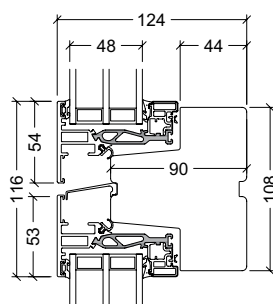
90mm tværpost
