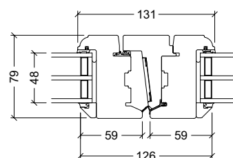
Anslag til 2-fløjet vindue og terrassedør (vinduesdør)
