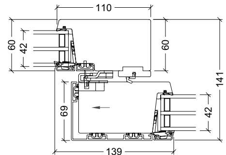
Lodpost, hæveskydedør
