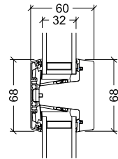
68mm gennemgående sprosse, 2-lags rude
