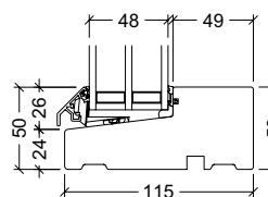
Bundkarm
