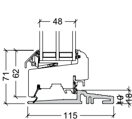
18mm HELO® bundkarm, terrassedør (vinduesdør) OBS: 22,5mm ved 148mm karm
