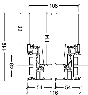
114mm lodpost (tværpost)
