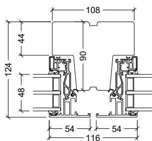
90mm lodpost (kun til vinduer)
