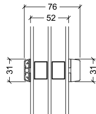
31mm energisprosse, 3-lags rude
