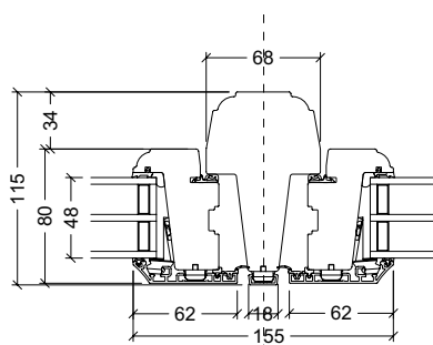
Lodpost, gående rammer Fast eller gående post
