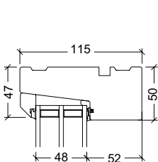
Overkarm
