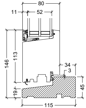
45mm hårdtræsbundkarm, udadgående dør
