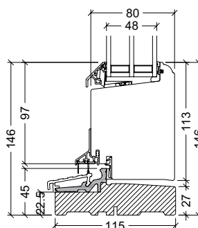
45mm hårdtræsbundkarm, indadgående dør
