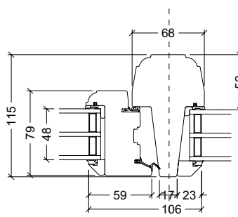
Kombinationslodpost
