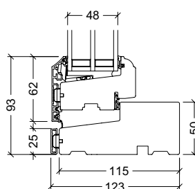
Bundkarm, gående ramme samt fastskruet ramme
