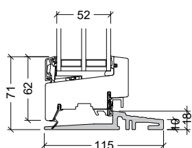
18mm HELO® bundkarm, terrasedør (vinduesdør) OBS: 22,5mm ved dyb karm
