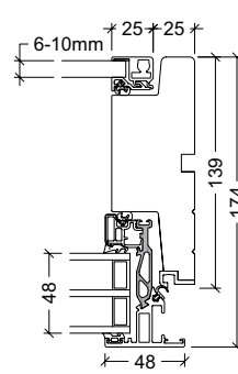
139mm karm med forsatsramme til vendevindue med 48mm rammeprofil
