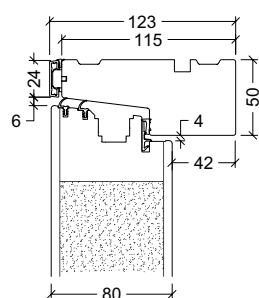
Overkarm
