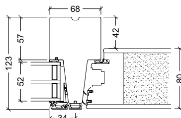
Lodpost til fast sideparti
