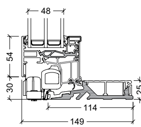
25mm bundkarm m/alu- slidskinne, skydedør
