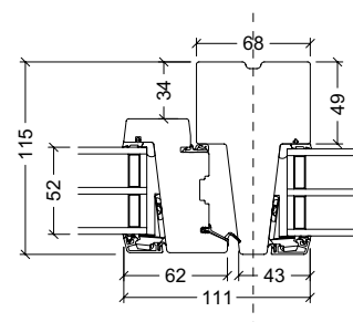
Kombinationslodpost
