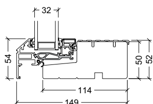
52mm bundkarm m/alu-slidskinne, terrasedør
