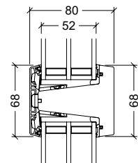
68mm gennemgående sprosse, 3-lags rude
