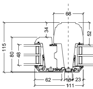
Kombinationslodpost
