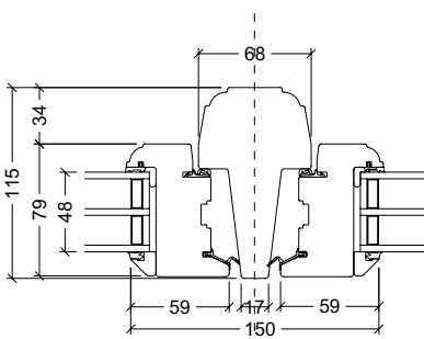
Lodpost, gående rammer Fast eller gående post
