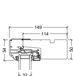
Overkarm
