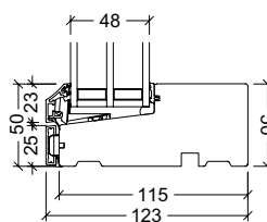
Bundkarm
