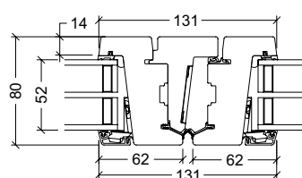
Anslag til 2-fløjet vindue eller terrasedør (vinduesdør)
