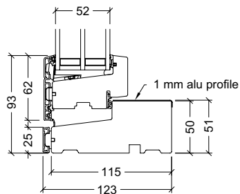
50mm bundkarm med alu-slidskinne, terrasedør (vinduesdør)
