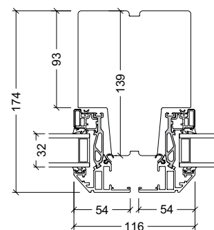
139mm lodpost (tværpost)
