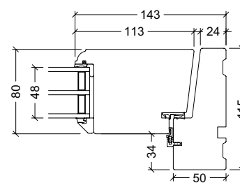
Sidekarm VELFAC Classic trædør
