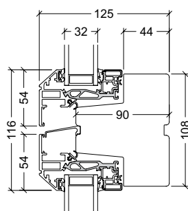
90mm tværpost
