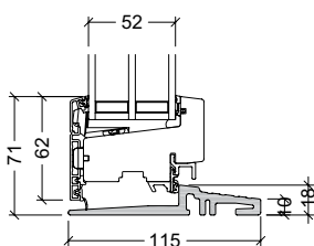
18mm HELO® bundkarm, terrasedør (vinduesdør) OBS: 22,5mm ved 148mm karm
