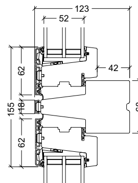
Tværpst, gående rammer
