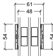
54mm energisprosse 3-lags rude
